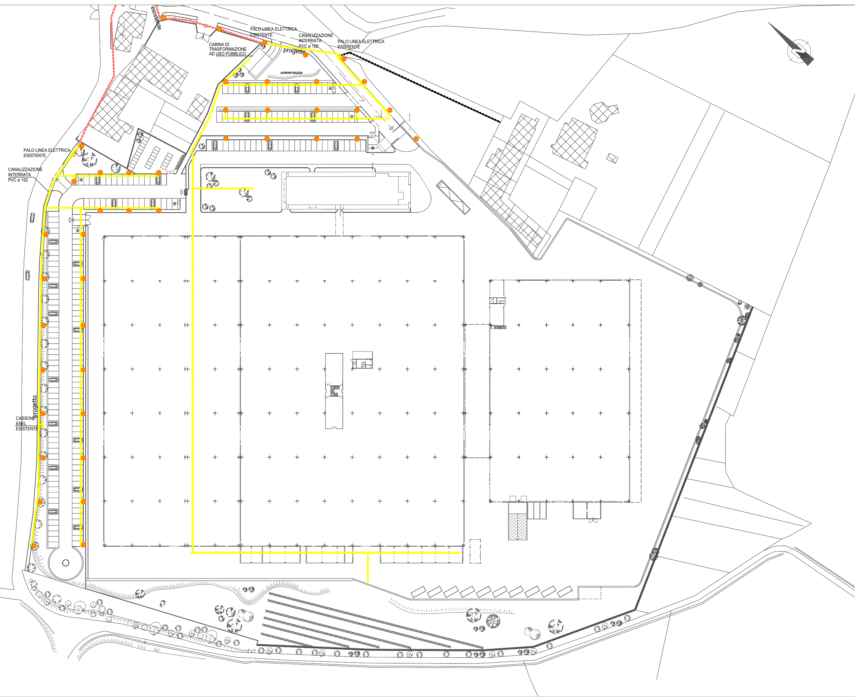
PLANIMETRIA RETE ELETTRICA REALIZZATA COME DA PEC APPROVATO
