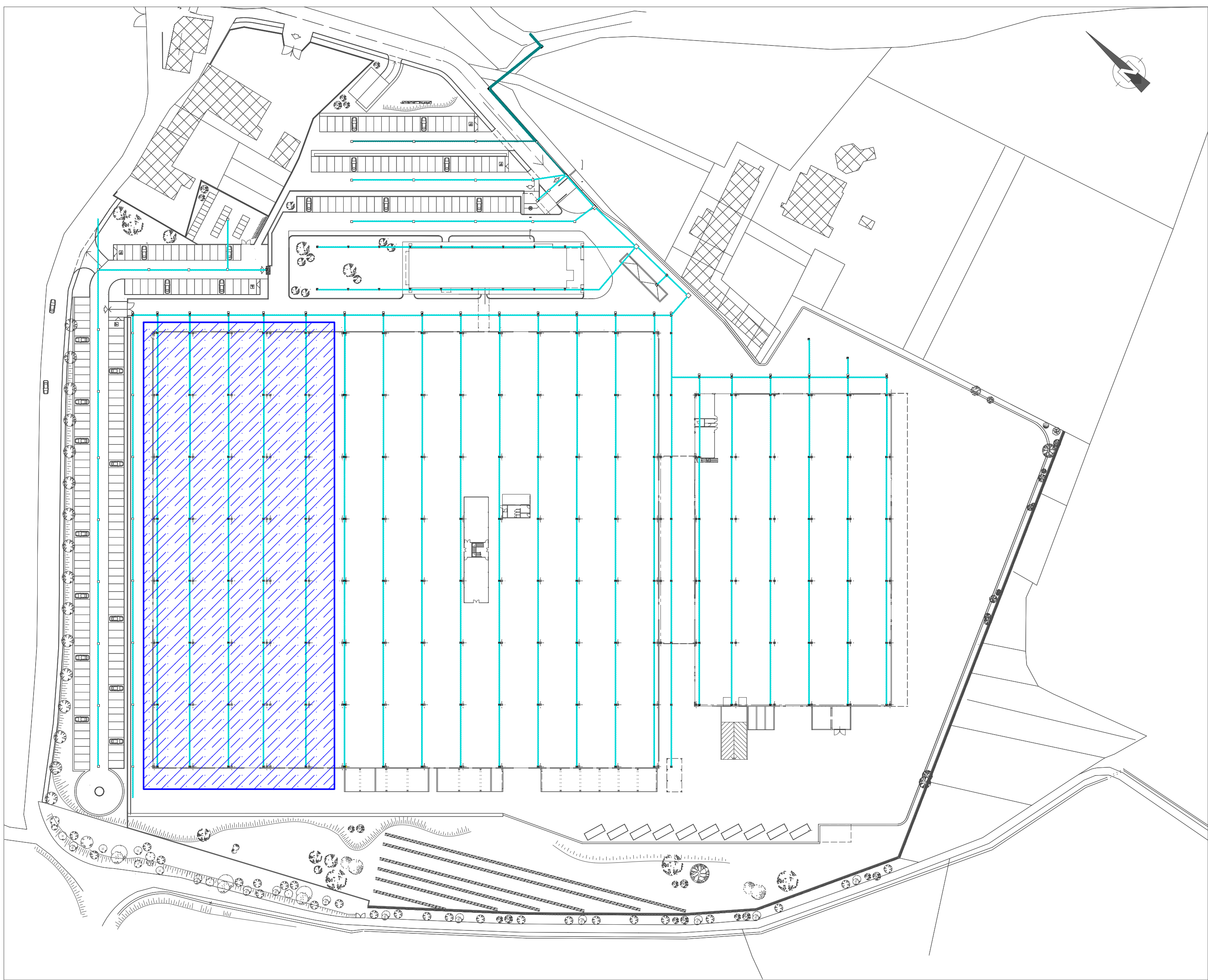
PLANIMETRIA RACCOLTA ACQUE METEORICHE COME DA PEC APPROVATO
