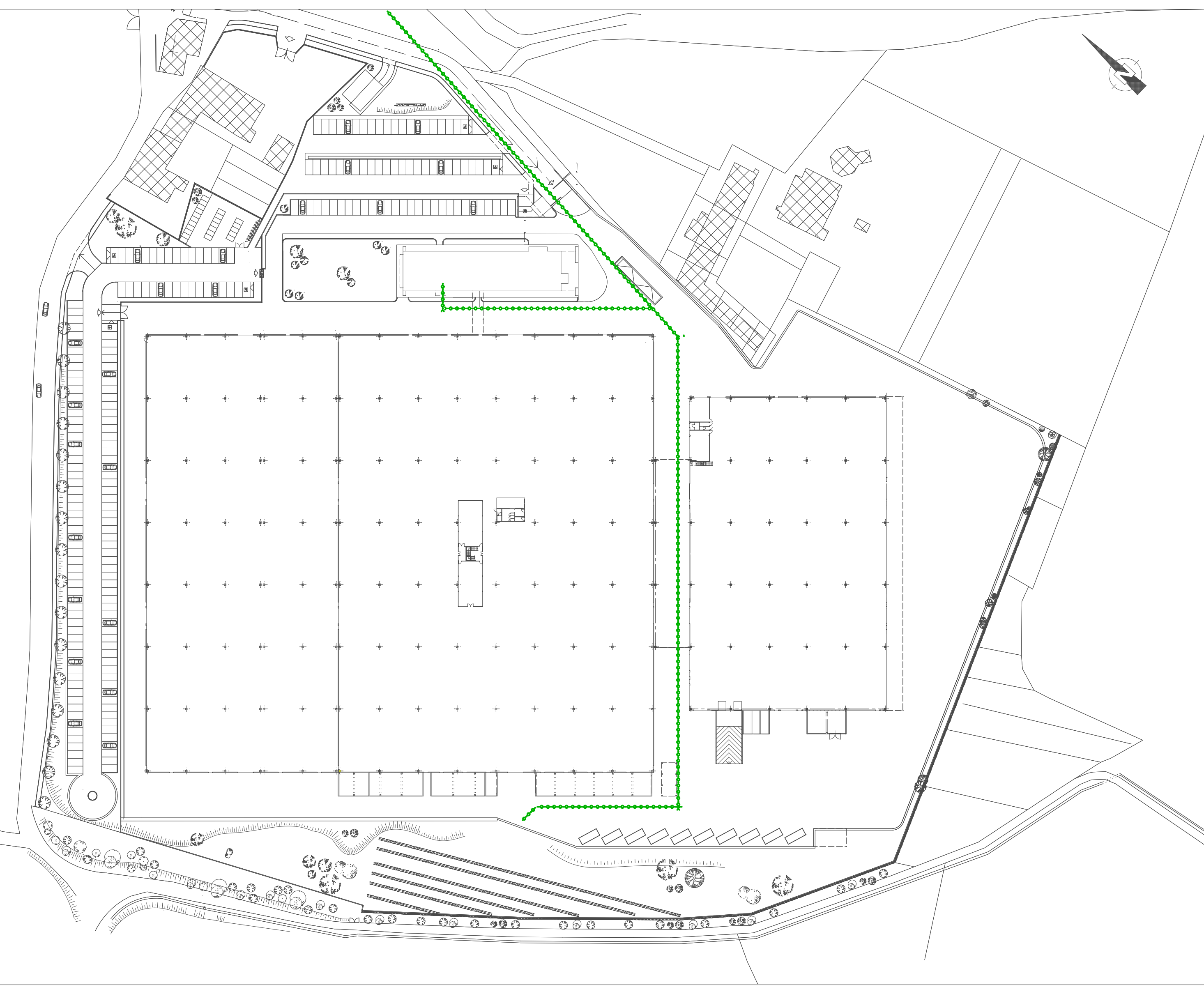
PLANIMETRIA RETE METANO REALIZZATA COME DA PEC APPROVATO
