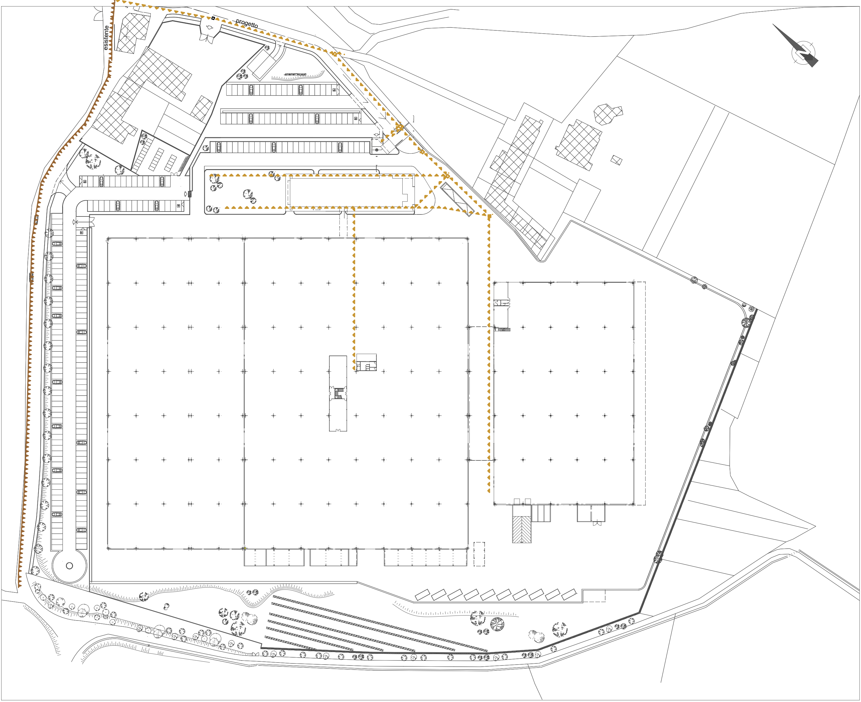
PLANIMETRIA RETE FOGNARIA
