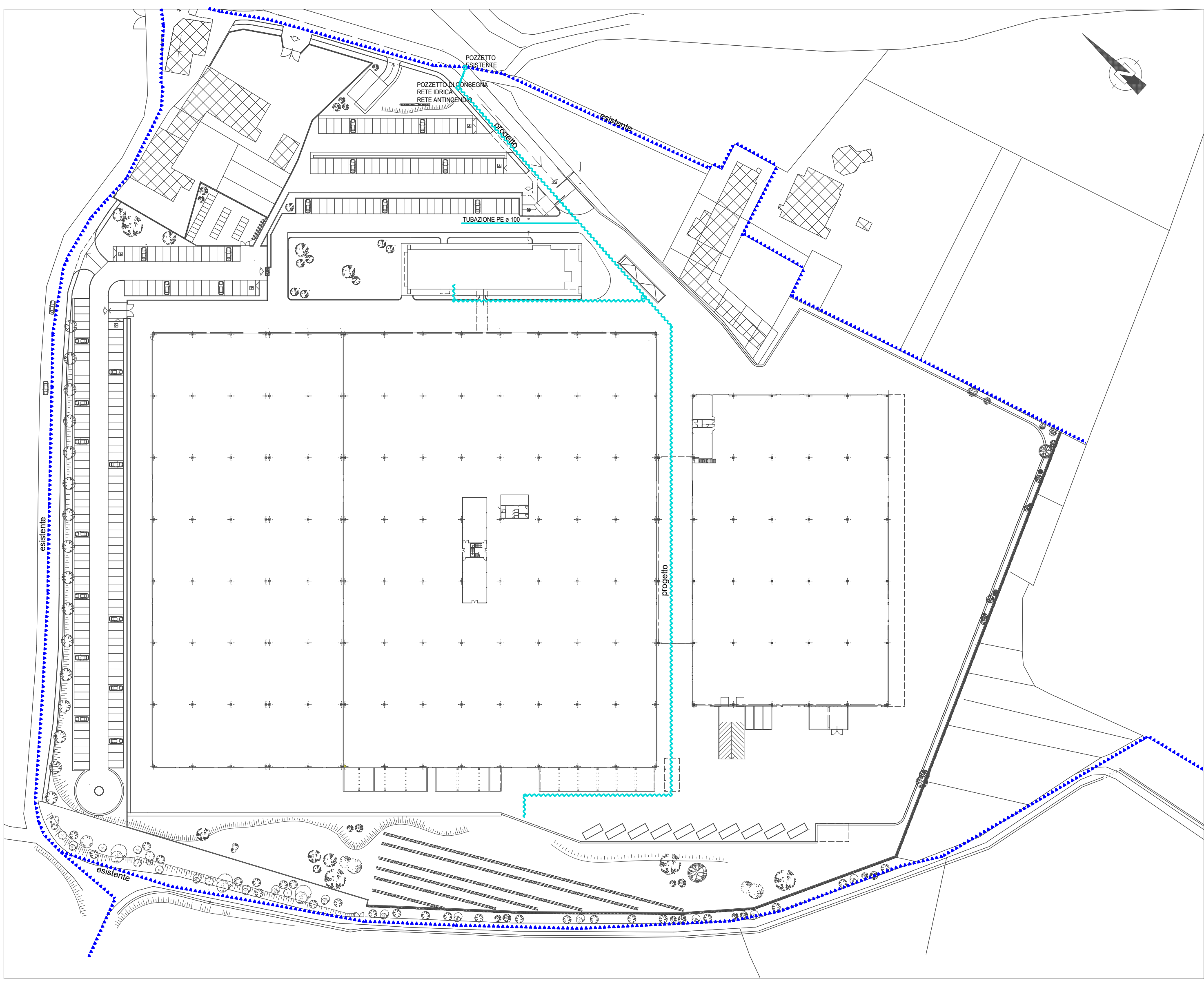
PLANIMETRIA DISTRIBUZIONE RETE IDRICA REALIZZATA COME DA PEC APPROVATO
